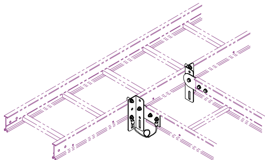
接続パターンB
