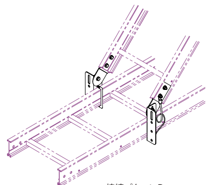
接続パターンD
