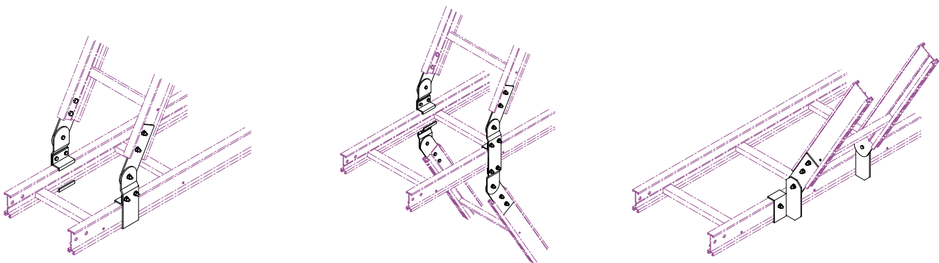
垂直分岐自在金具 型番 (21) (販売単位：1 組／両側)
