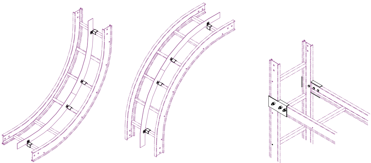
UP・DN用 セパレーター&固定金具 (注) 固定金具材質：SUS304 (販売単位：1 個)
