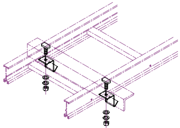
アングルサポート取付金具 型番 (48) (販売単位：1 組／両側)
