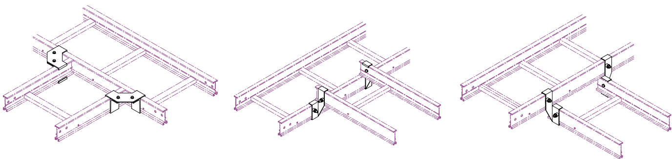
水平分岐金具 型番 (43) (販売単位：1 組／両側)
