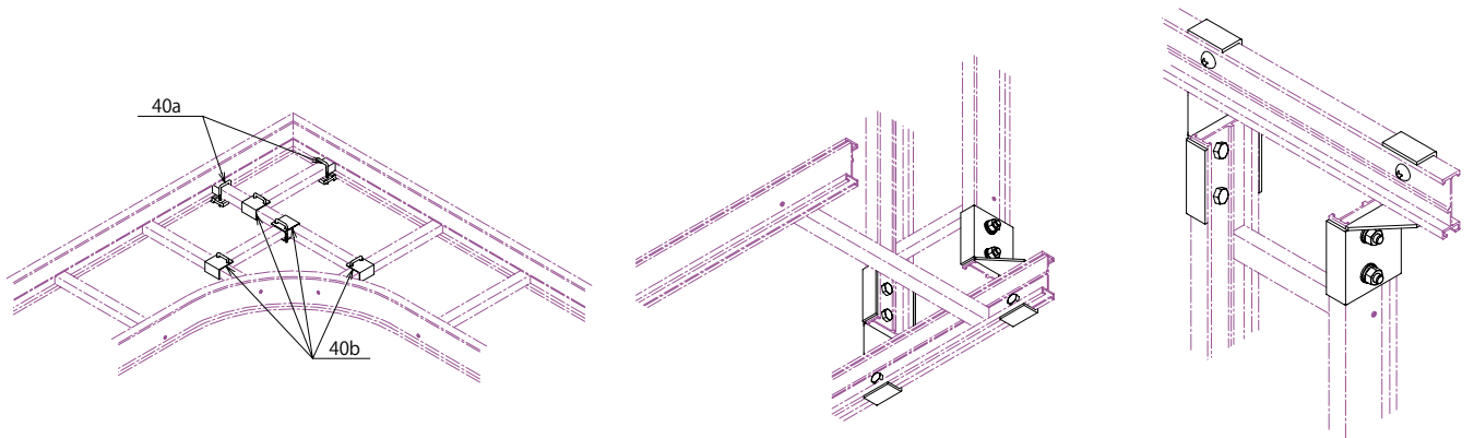
子桁取付金具 型番 (40a&40b) (注) 材質：SUS304 (販売単位：1 個)
