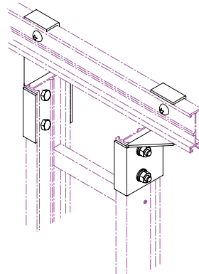
垂直立下げ金具 型番 (42) (販売単位：1組／両側)
