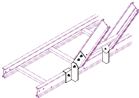
側面垂直分岐自在金具a 型番 (23) (販売単位：1組／両側)
