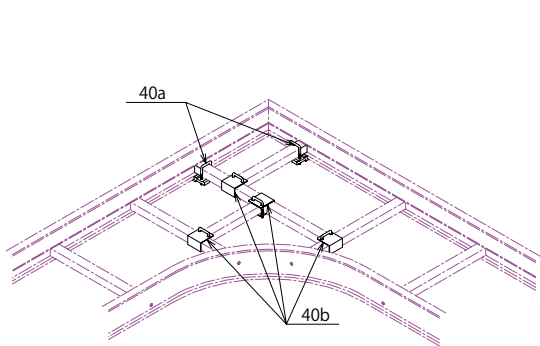
子桁取付金具 型番 (40a&40b) (注) 材質：SUS304 (販売単位：1個)
