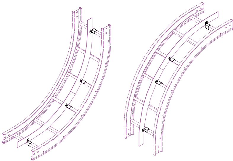
UP・DN用 セパレーター&固定金具 (注) 固定金具材質：SUS304 (販売単位：1個)
