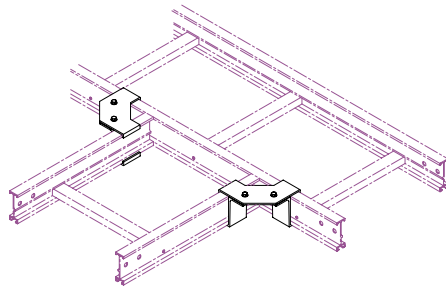
水平分岐金具 型番 (43) (販売単位：1組／両側)
