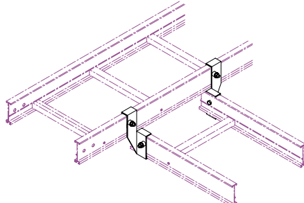
側面分岐金具b 型番 (45) (販売単位：1組／両側)
