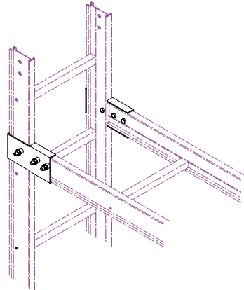
垂直分岐金具 型番 (22) (販売単位：1個／両側)
