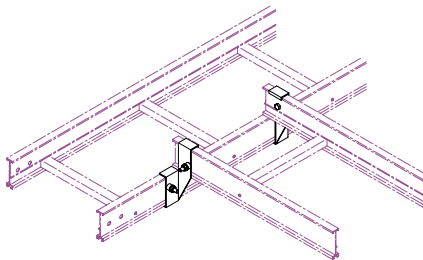
側面分岐金具a 型番 (44) (販売単位：1組／両側)
