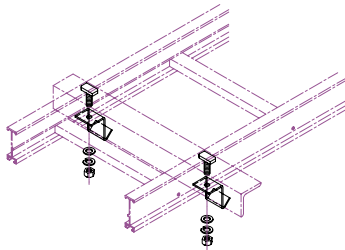
アングルサポート取付金具 型番 (48) (販売単位：1組／両側)
