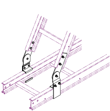
垂直分岐自在金具 型番 (21) (販売単位：1組／両側)
