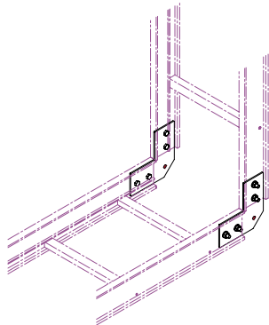
直角取付金具 型番 (47) (販売単位：1組／両側)
