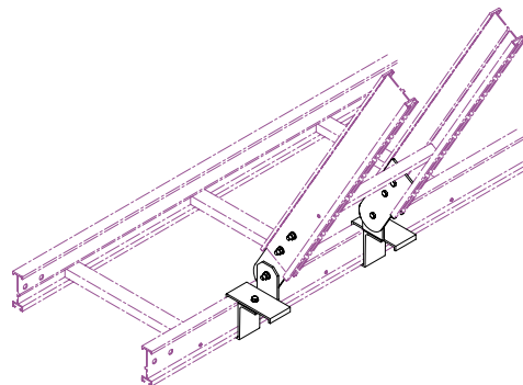
側面分岐自在金具 型番 (46) (販売単位：1組／両側)
