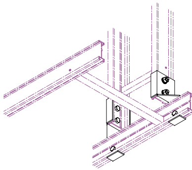
垂直立上げ金具 型番 (41) (販売単位：1組／両側)
