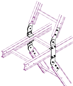
垂直分岐自在金具 型番 (21a) (販売単位：1組／両側)
