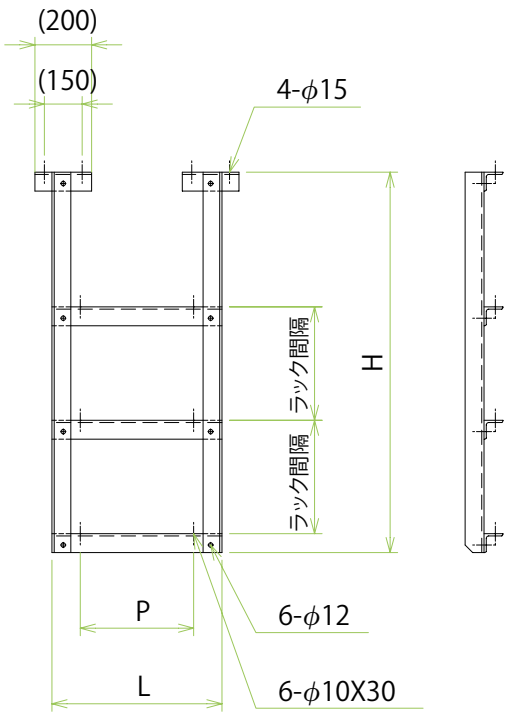
この図は 3段の場合を示しています。
