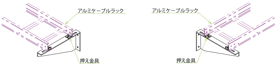
押え金具使用の場合
