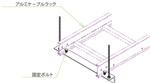
固定ボルト使用の場合
